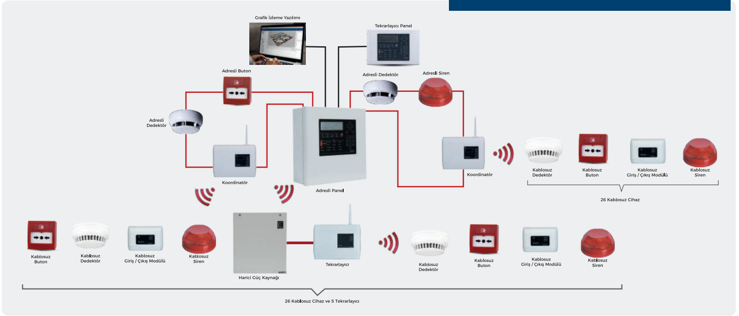
Kablosuz Adresli Yangın Sistem Şeması
